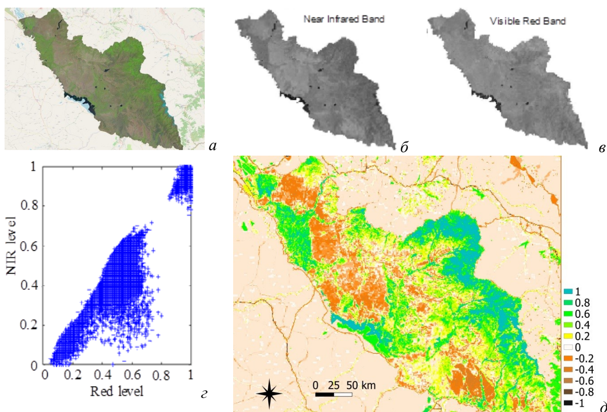
Рис. 3. Поэтапное построение тематической карты вегетационного индекса: а - цветовые преобразования; б, в - выделение NIR и RED изображений; г - анализ двумерного пространства спектральных признаков; д - карта распределения вегетационного индекса NDVI.
