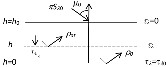
Рис. 1. Схема рассеяния света в атмосфере
