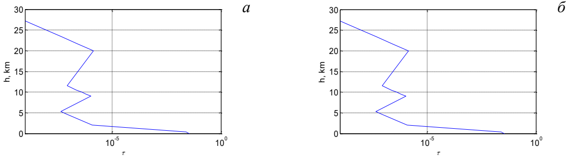
Рис. 2. Вертикальные профили оптической толщины атмосферы \tau(h) : а-по данным снимка LC08_L1TP_169033_20240715_20240715_02_RT_B4, б-по данным снимка LC08_L1TP_169033_20240715_20240715_02_RT_B5.
