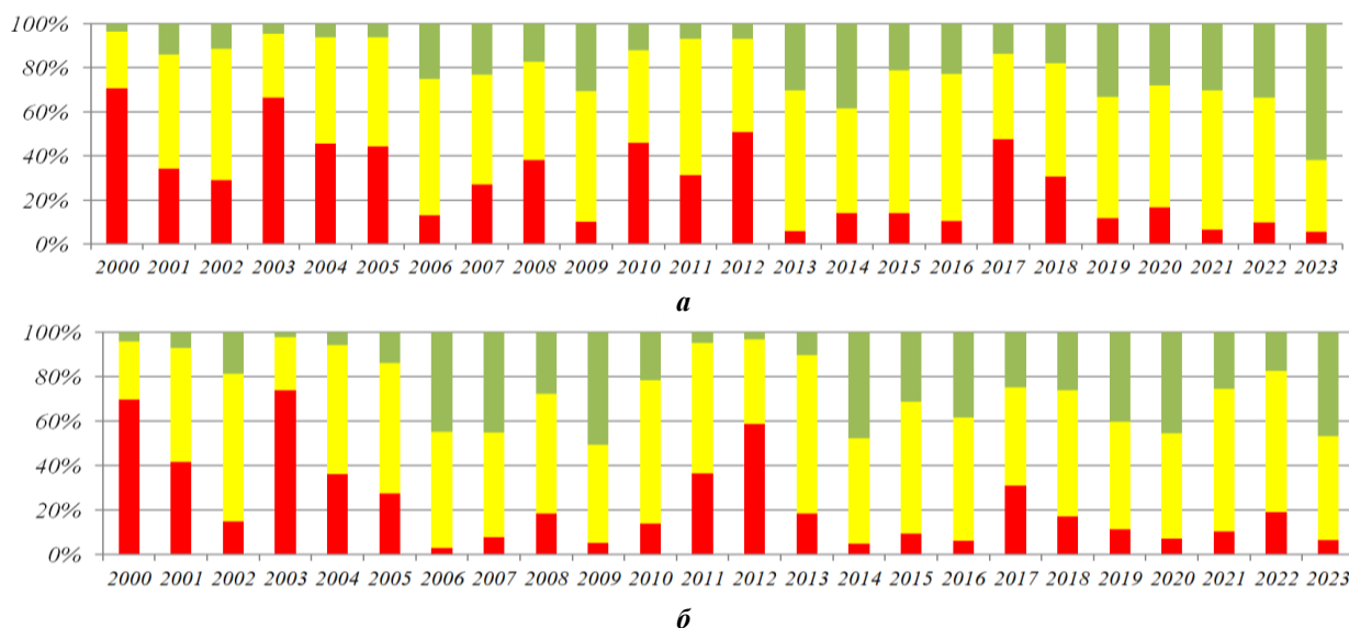
Рис. 5. Соотношение площадей классов хвойных (а) и лиственных (б) лесов с разными значениями IVCI для территории пяти районов Костромского Заволжья
