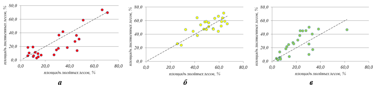
Рис. 6. Соотношение площадей классов хвойных и лиственных лесов с разными значениями IVCI для территории пяти районов Костромского Заволжья: класс индекса «стресс» (а), «среднее» (б), «рост продуктивности» (в)
