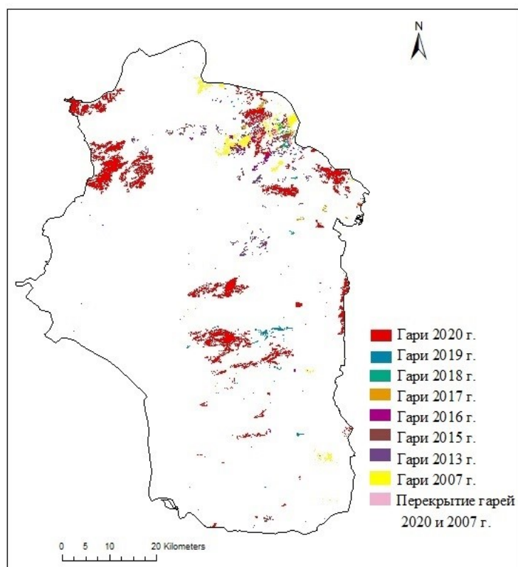
Рис. 7. Распределение гарей 2007, 2013, 2015-2020 гг. на территории САР
