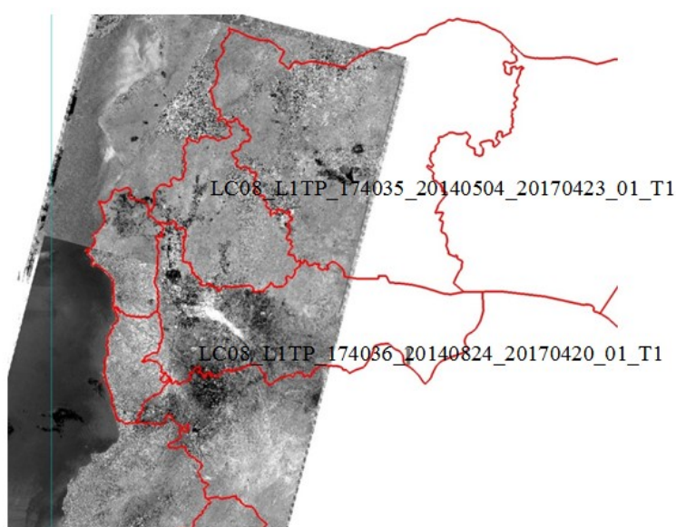
Рис. 2. Покрытие снимками Landsat 2014 г. территории исследования
