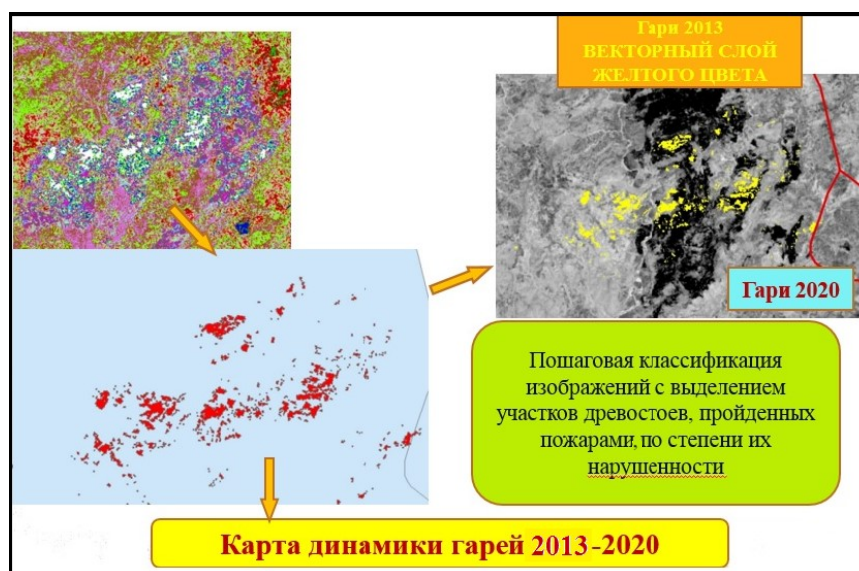
Рис. 5. Тематическое картографирование гарей за разные годы
