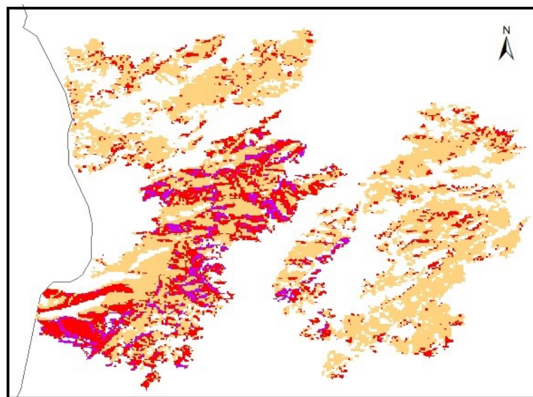
Рис. 6. Фрагмент тематического слоя «Гари 2020» на территории мухафаза Латакия (САР), содержащий три класса наземного покрова по степени поражения огнем (нет легенды)
