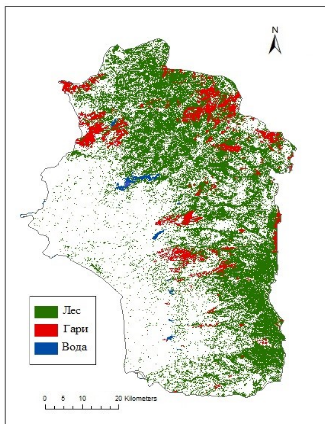
Рис. 8. Распределение площадей гарей за исследуемый период на территории мухафаза Латакия САР
