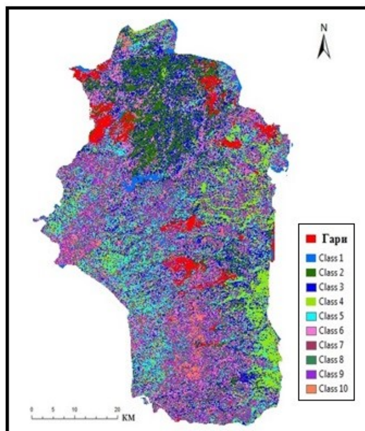
Рис. 4. Карта мухафаза Латакия, полученная с помощью пошаговой классификации ISODATA. Класс гари 2020 г. выделен красным цветом
