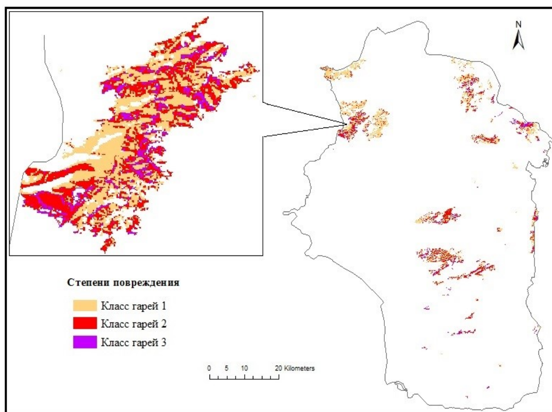
Рис. 9. Степень повреждения на лесных гарях в результате пожаров 2020 г. на территории мухафаза Латакия САР
